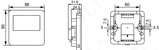
Габаритні розміри
