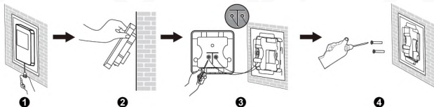
Етапи розбирання
