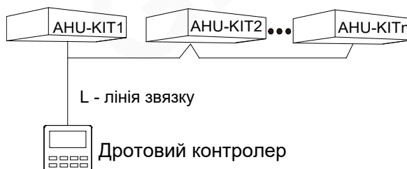
Мал.3.2 Один дротовий контролер до кількох АНУ-KIT
