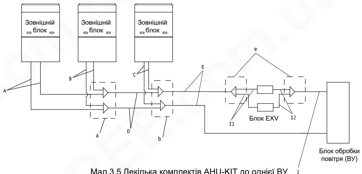
Мал.3.5 Декілька комплектів АНУ-KIT до однієї ВУ
