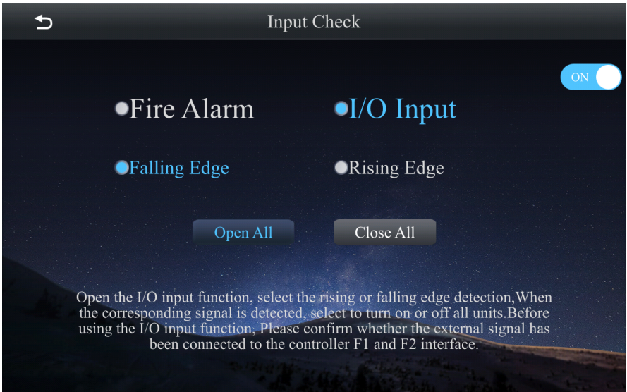
Fig. 5.16 IO input page
