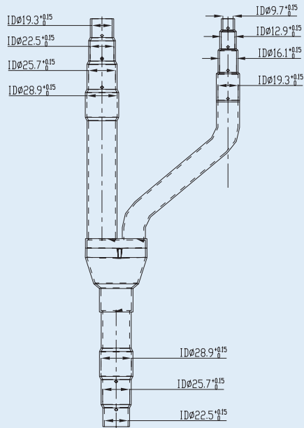
Газовая труба низкого давления
