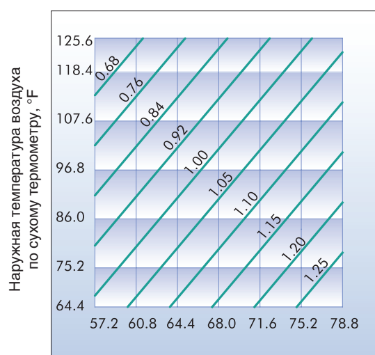
Наружная температура воздуха по влажному термометру, °F
