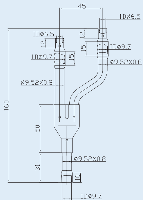
Жидкостная труба
