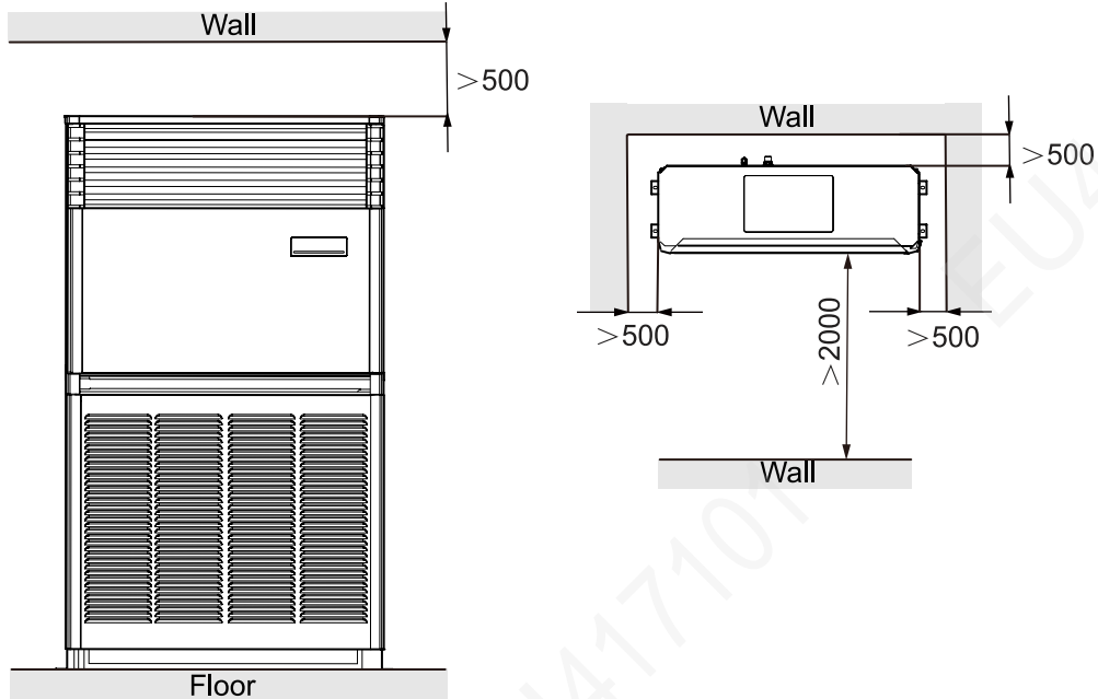
GMV-N280L/A-D
