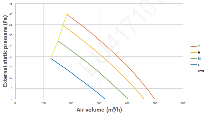
GMV-ND22ZA/A-T GMV-ND28ZA/A-T
